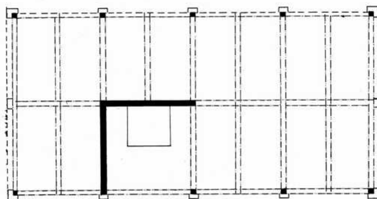
6. A 7. ÚROVEŇ
