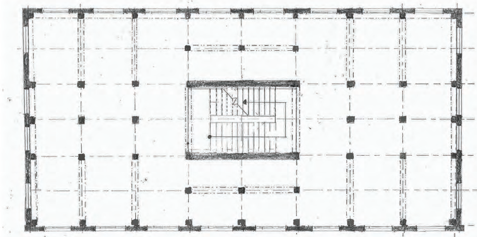
PODLAŽÍ 1
