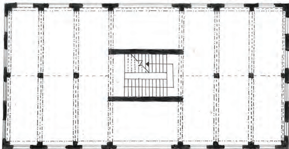
PODLAŽÍ 6
