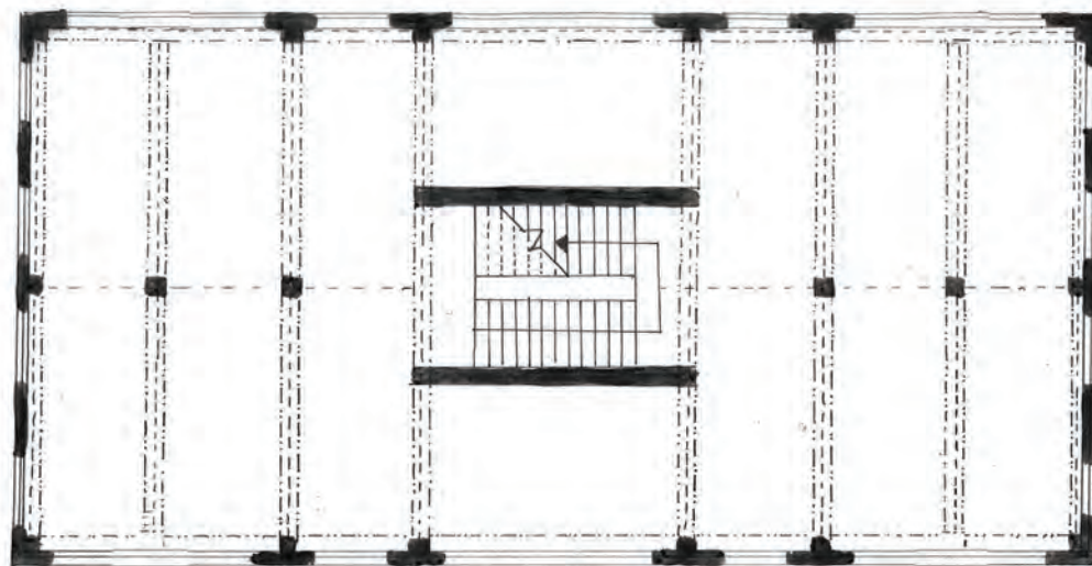
PODLAŽÍ 7
