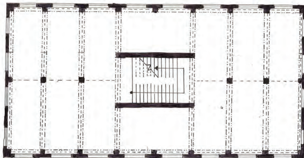
PODLAŽÍ 3 - 5
